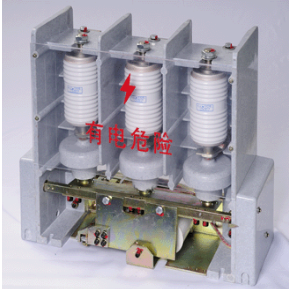
JCZ5-400A/12kV-S型(机械保持)交流真空接触器
